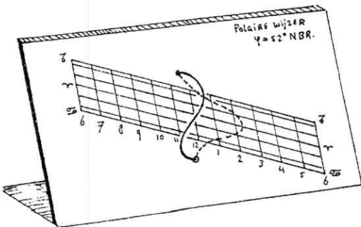
Fig. 10. Monofilaire zonnwijzer met rechte homogene uurlijnen en rechte, evenwijdige datumlijnen, van Willem Bits. De schaduwgever is een draad die zich als een driedimensionale S over het tafereel slingert.
