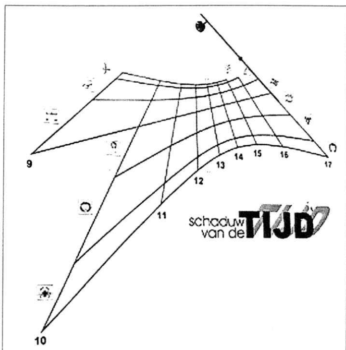
Verticale west afwijkende zonnewijzer van W. Leenders.
