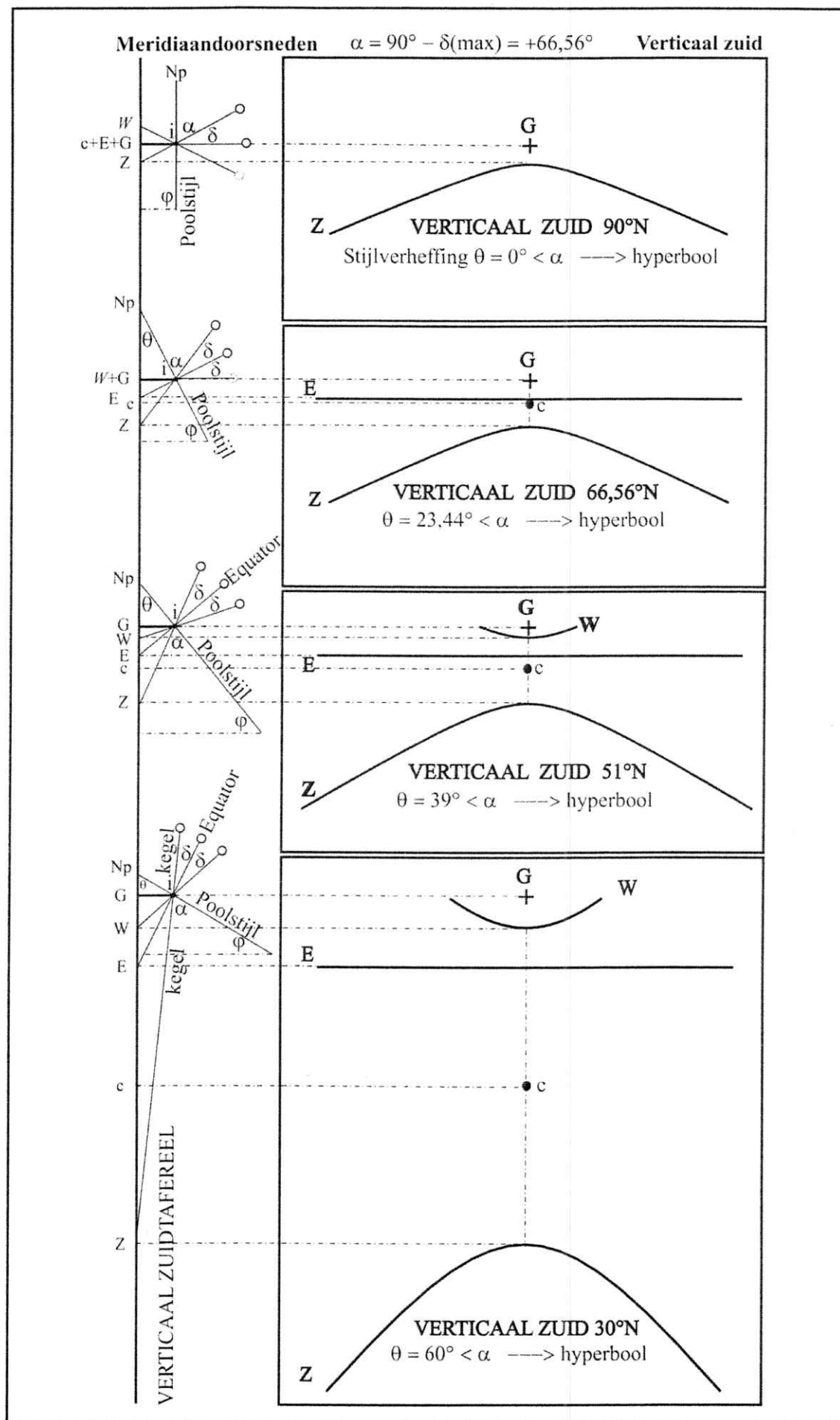
Fig. 8: evolutie van de hyperbolen op een verticaal zuidafereel op verschillende breedten (noordelijk halfrond).
