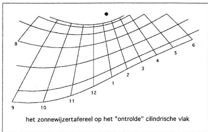
Fig. 10: 'ontrolde' cilindervlak.
